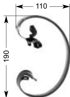
25 027 0,19 kg □ 12 x 5 mm
