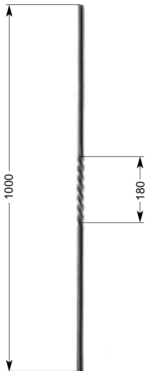
31 603 0,97 kg □ 12 x 12 mm
