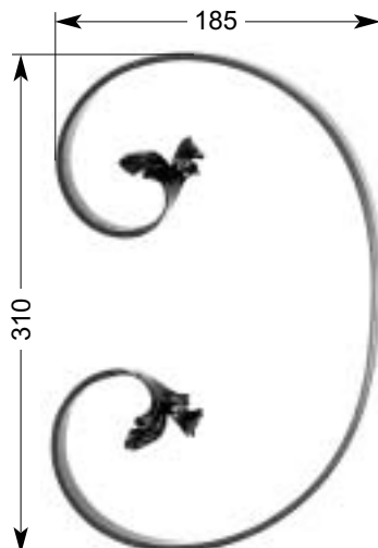
25 001 0,42 kg □ 12 x 5 mm
