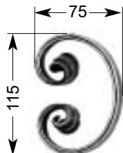
25 003 0,18 kg □ 12 x 5 mm
