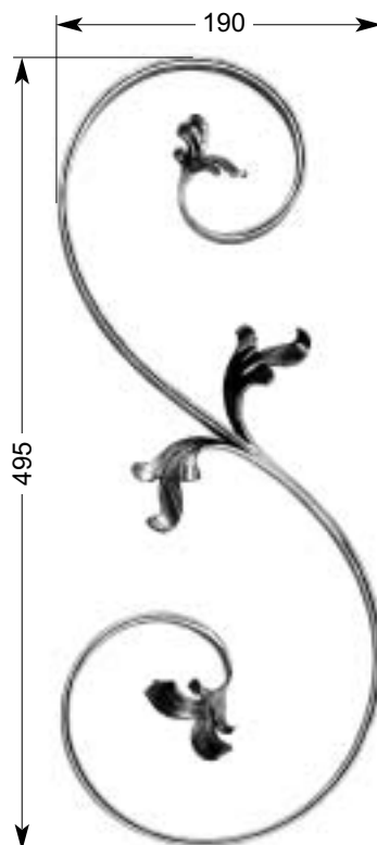
25 062 0,67 kg □ 12 x 5 mm
