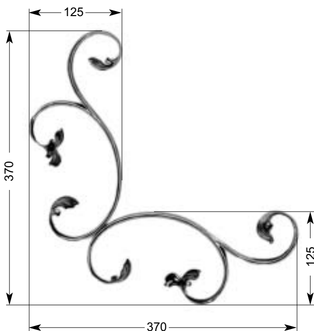
25 170 0,58 kg □ 12 x 5 mm
