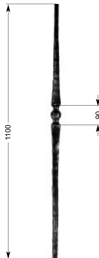
30 512 Anfangsstab Endpost Balustre de départ 6,19 kg □ 25 x 25 mm
