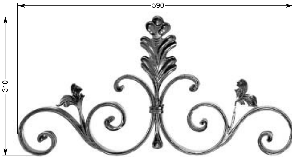
25 371 2,48 kg □ 16 x 8 mm Aufsatzverzierung Ornamental top Couronnement décoratif
