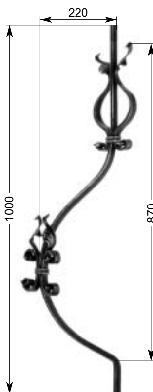
32 602 Korbstab Convex grille bar Barreaux de grille en anse-de-panier 2,50 kg □ 16 x 8 mm
