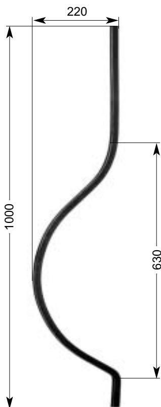
32 601 Korbstab Convex grille bar Barreaux de grille en anse-de-panier 1,13 kg □ 16 x 8 mm
