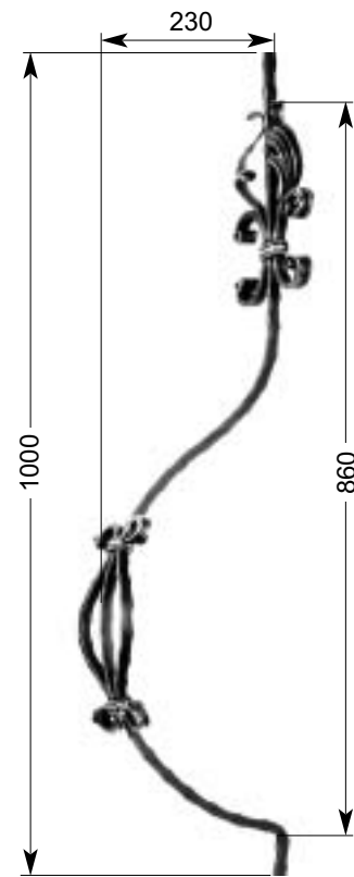
32 402 Korbstab Convex grille bar Barreaux de grille en anse-de-panier 2,76 kg □ 16 x 8 mm
