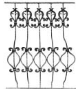
32 402 Korbstab Convex grille bar Barreaux de grille en anse-de-panier 2,76 kg □ 16 x 8 mm
