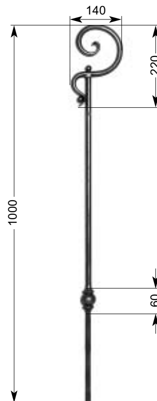
35 630 1,91 kg Ø 14 mm
